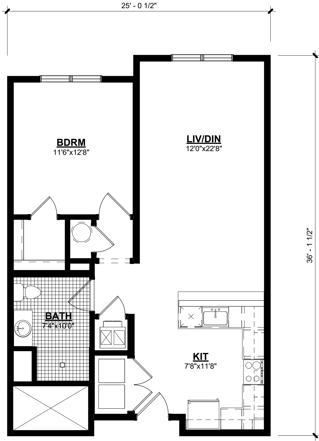
Unit 1B Scale: 3/16" = 1'-0"
